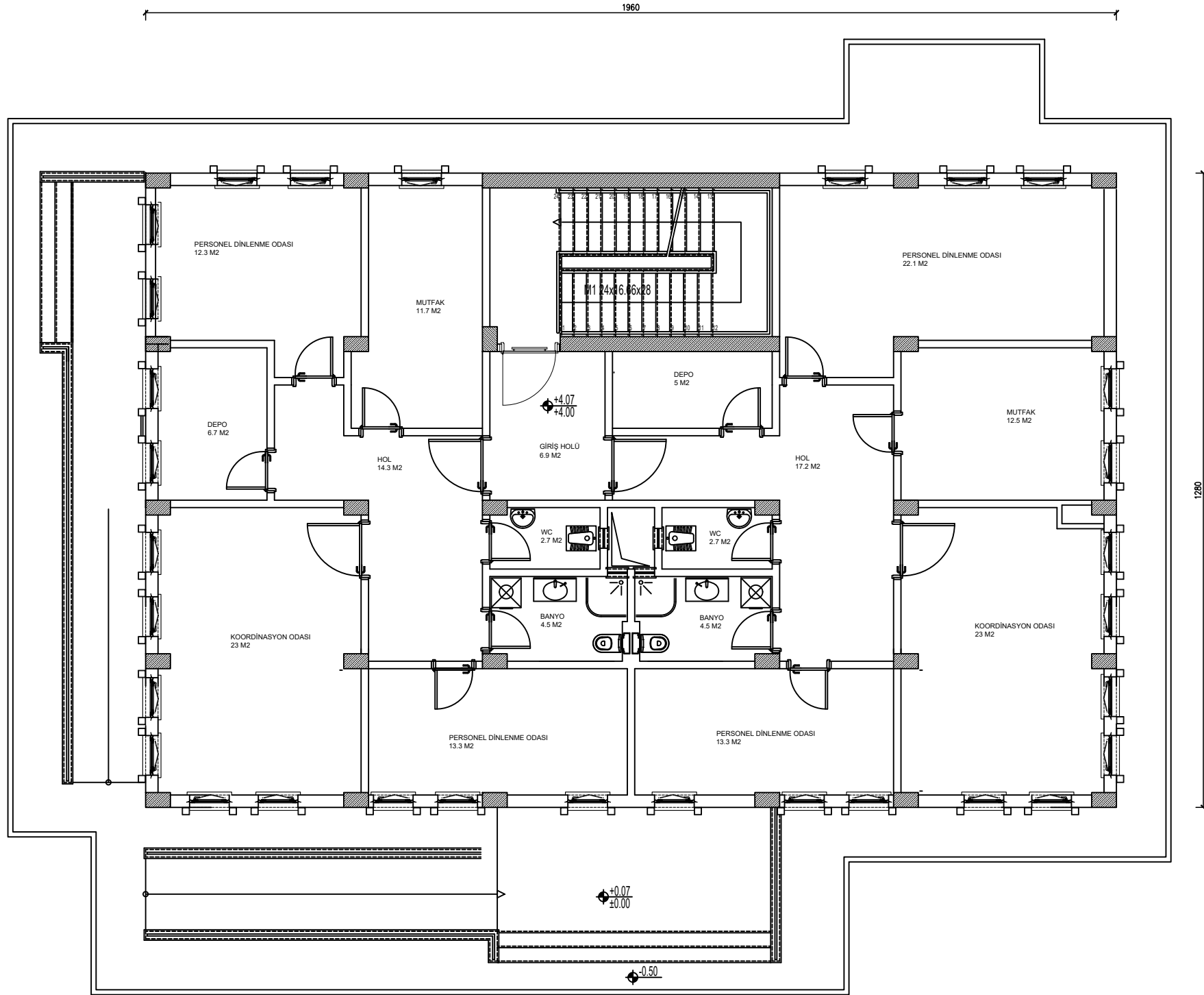
2 HEKİMLİ AİLE SAĞLIĞI MERKEZİ VE 112 ACİL SAĞLIK HİZMETLERİ İSTASYONU 1. KAT PLANI ALAN:250 M 2
