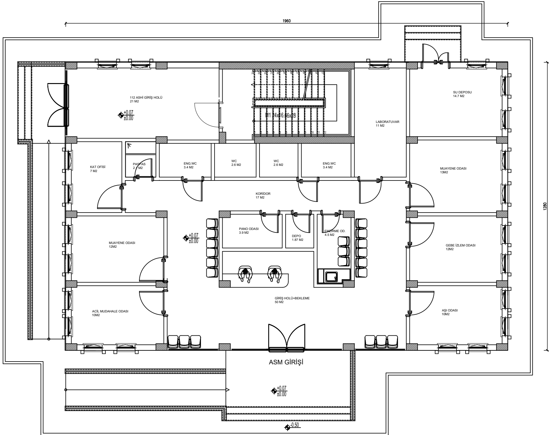
2 HEKİMLİ AİLE SAĞLIĞI MERKEZİ VE 112 ACİL SAĞLIK HİZMETLERİ İSTASYONU ZEMİN KAT PLANI ALAN:250 M2
