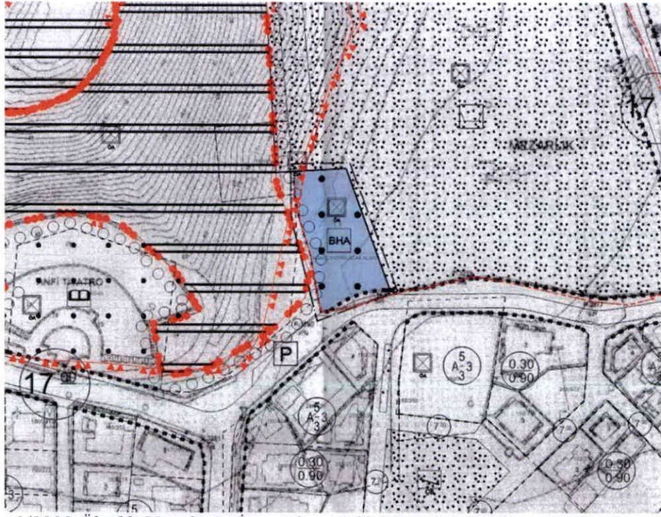
1/1000 Ölçekli Uygulama İmar Planı Teklifi 287 Ada 43 Parselin Bir Kısım
