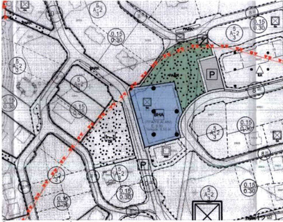
1/1000 Ölçekli Uygulama İmar Planı Teklifi 326 Ada 1 Parsel ile 327 Ada 1 Parsel ve çevresi
