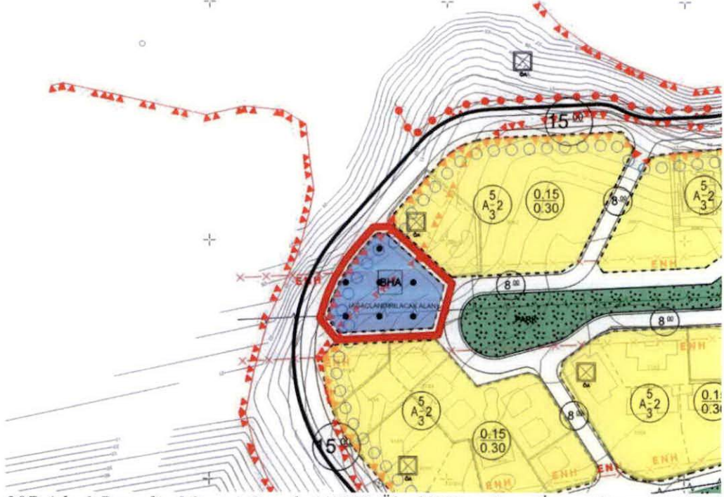
307 Ada 1 Parselin Mevcut Onaylı 1/1000 Ölçekli Uygulama İmar Planındaki Yeri
